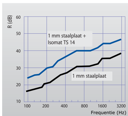
Verbetering van de luchtgeluidisolatiewaarde R van Isomat TS als functie van de frequentie, gemeten volgens DIN 52210
